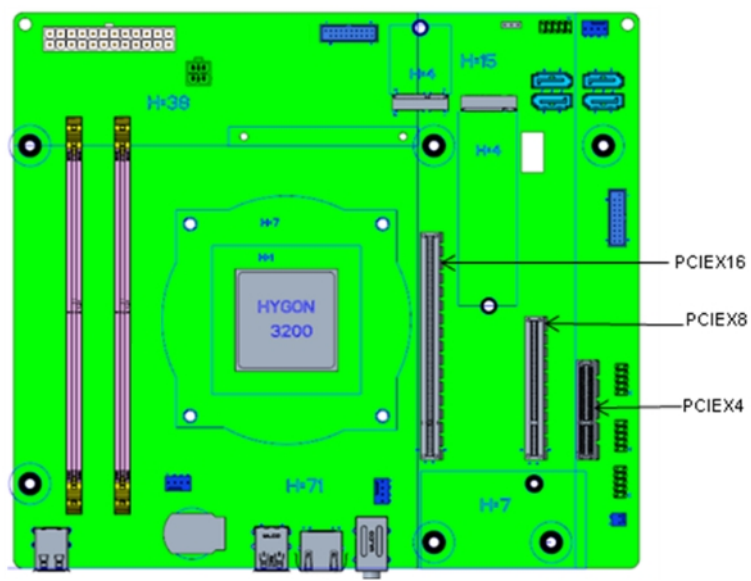
图示为主板支持标准的PCIEX16（显卡）、PCIEX8（专有SOC配置X1信号，通用配置支持X2信号）、PCIEX4接口。
