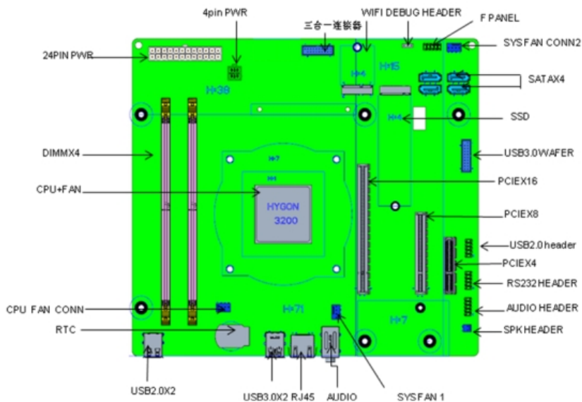
GM9-5001 接口位置图
