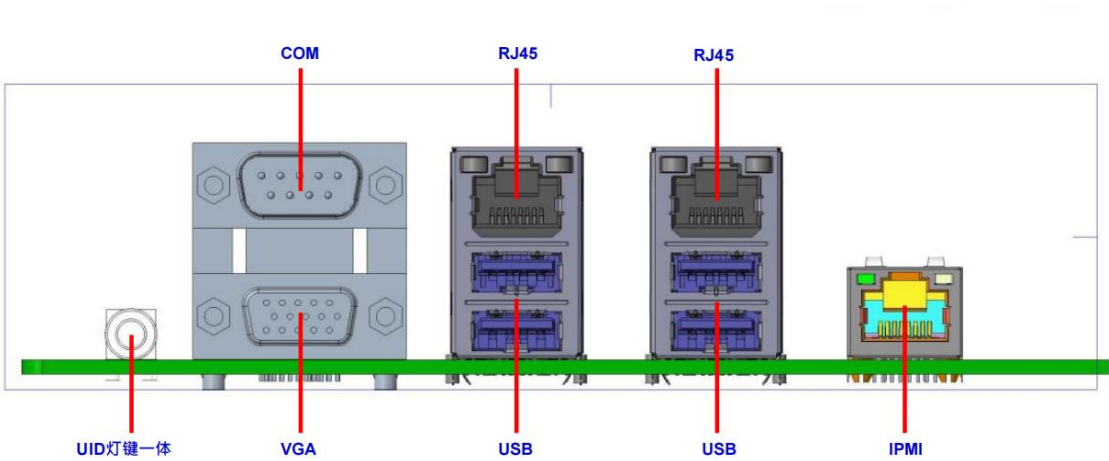
图 5 产品后视图
