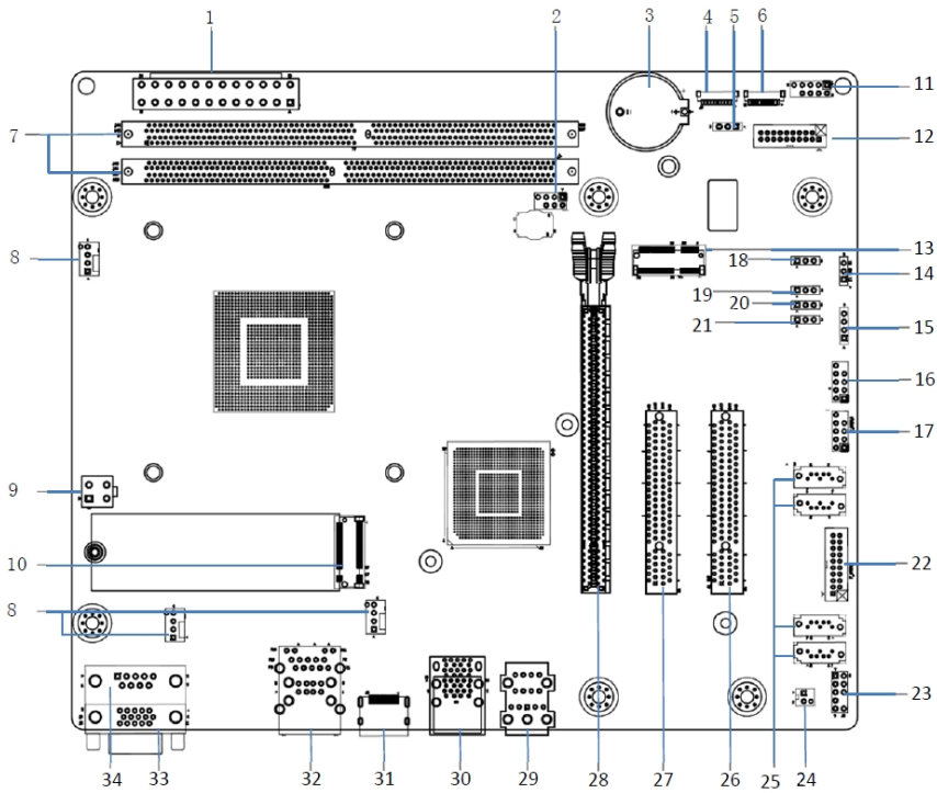
接口位置图
