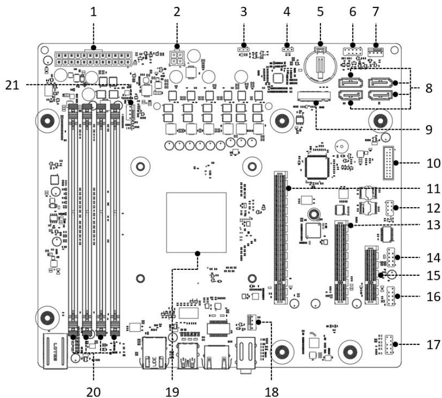
GM9-5002-01接口位置图
