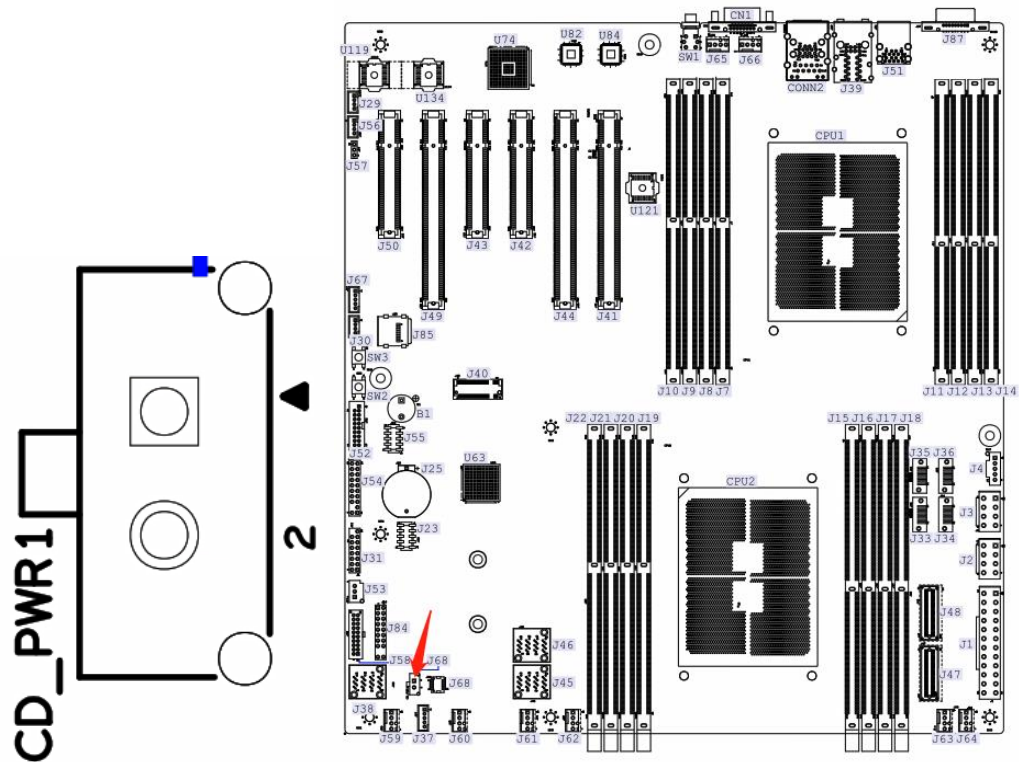
PIN 定义:
