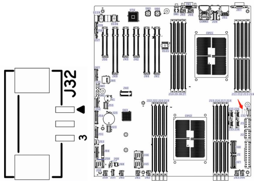
PIN 定义:
