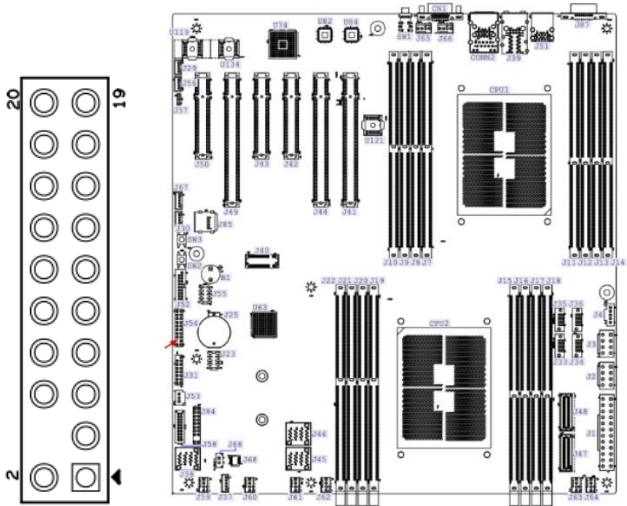
PIN 定义:
